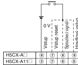
V činnosti při sepnutém relé
