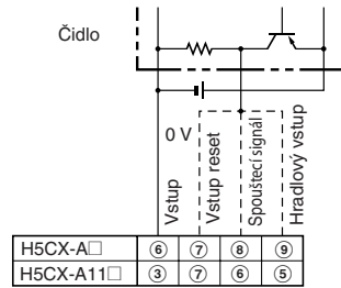
V činnosti při zapnutém tranzistoru
