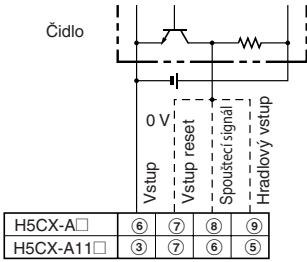
V činnosti při vypnutém tranzistoru
